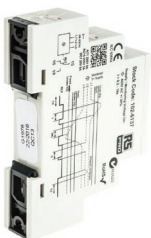
Releu de monitorizare a tensiunii, cu o ieșire SPDT de 8A, trifazat, montare pe șină DIN.
